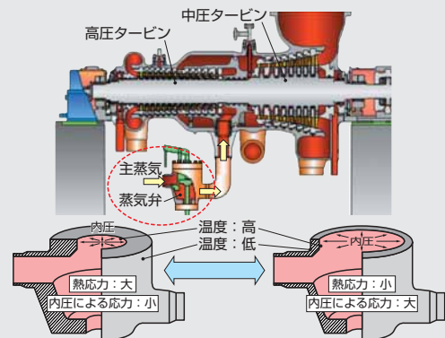
図2. 構造物形状と応力の関係 (蒸気弁の例) — 蒸気弁は、タービンの蒸気入口部に配置され、発電量に応じて高温蒸気の流量を制御します。この部品の肉厚が厚いと、内圧による応力は小さいが熱応力が大きくなり、肉厚が薄いとその逆になります。形状最適化手法により、これらの応力の和が最小となる構造を求めることができます。
