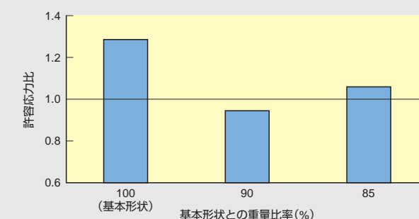
図5. 形状最適化後の応力値 — 発生する応力を許容応力以下に抑えるとともに、重量を10%低減できる形状を達成することができました。
