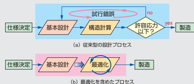
図1. 製品開発における強度設計プロセス — 従来設計プロセスは繰り返し試行錯誤が必要でしたが、最適化プロセスでは短時間に最適解を得られます。
