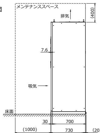
右側面図
