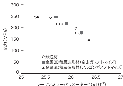
図3. 金属3D積層造形材（12Cr鋼）のクリープ特性
